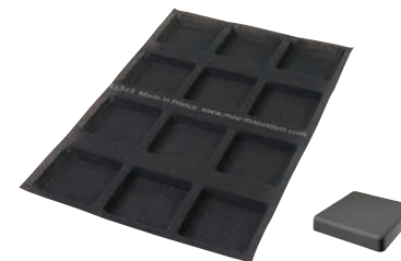
④ スクエア 12取 011343-4060 <WMA-20> 1-1122-0401 ¥18,700 600×400 出来上がり寸法:110×110×H20
