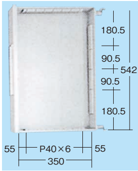
■仕切り寸法
