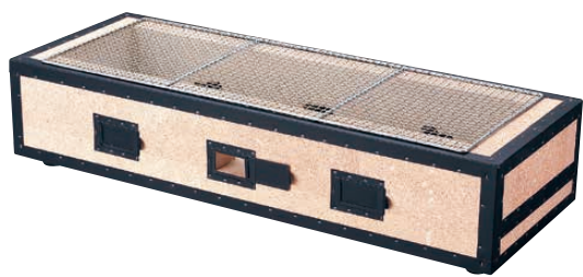
① 炭火バーベキューコンロ BQ-22号 (8~12人用) 〈DBC-39〉B 1-0773-0101 ¥86,000 920×350×H200 質量25kg 付属品:焼アミ1枚 材質:けいそう土
