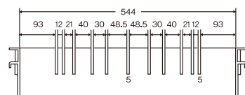
⑭ PPコンテナ PC-37B用仕切り板 〈AKV-Q2〉 1-0156-1401 大 555×180×厚さ5 ¥1,210 1-0156-1402 小 355×180×厚さ5 ¥ 900 材質:ポリプロピレン
