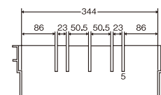
⑯ PPコンテナ PC-27B用仕切り板 〈AKV-Q0〉 1-0156-1601 大 555×130×厚さ5 ¥990 1-0156-1602 小 355×130×厚さ5 ¥770 材質:ポリプロピレン
