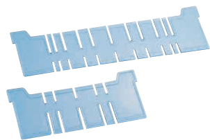
⑭ PPコンテナ PC-37B用仕切り板 〈AKV-Q2〉 1-0156-1401 大 555×180×厚さ5 ¥1,210 1-0156-1402 小 355×180×厚さ5 ¥ 900 材質:ポリプロピレン
