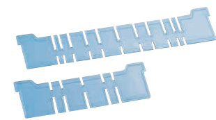
⑯ PPコンテナ PC-27B用仕切り板 〈AKV-Q0〉 1-0156-1601 大 555×130×厚さ5 ¥990 1-0156-1602 小 355×130×厚さ5 ¥770 材質:ポリプロピレン
