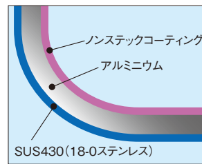
⑤ TKG IH セレクト 2層クラッド 両手 フライパン 〈PPE-14〉
