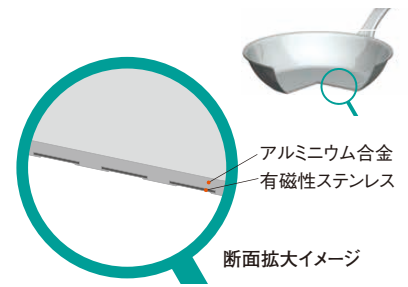
TKG IHキャストフライパン
