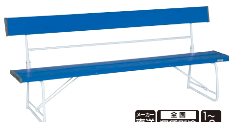
⑩ 折りたたみ式 背付ベンチ 1800 BC-300-018 青 〈UBV-08〉 1-2528-1001 ¥48,700 1,800×516×H740×座高370 材質:座面/硬質塩化ビニール 脚/スチールパイプに粉体塗装 背板縦サイズ:140mm 質量:約16.6kg ●座面両端は安全カバー付
