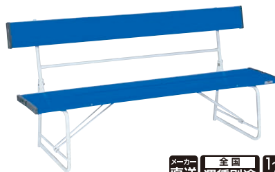
⑨ 折りたたみ式 背付ベンチ 1500 BC-300-015 青 〈UBV-07〉 1-2528-0901 ¥44,000 1,500×516×H740×座高370 材質:座面/硬質塩化ビニール 脚/スチールパイプに粉体塗装 背板縦サイズ:140mm 質量:約14.6kg ●座面両端は安全カバー付
