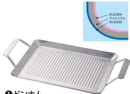
① ドンナム 三層鋼焼肉プレート 角型 (APL-61) 1-2156-0101 ¥16,000 kg 底面サイズ 412×236×H16 1.2 270×190 板厚: 3.0
