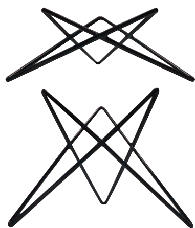
⑥ 3Dノンスリップスター 〈NNV-12〉B 1-1680-0601 M H100 ¥1,800 1-1680-0602 L H200 ¥2,500 材質:芯材/低炭素鋼 表面/PVCノンスリップ加工 上部175×底部260 ● 上部、底部どちらも使用可能で トレイやボール、大皿を安定して セッティング出来ます。
