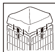
⑨ ワイヤーバスケット 〈KBS-01〉 1-1420-0901 大(90ℓ用) ¥9,600 400×400×H630 3.1kg 1-1420-0902 小(70ℓ用) ¥8,100 340×340×H606 2.5kg 材質:スチール線材にビニールコーティング ●折りたたみ式
