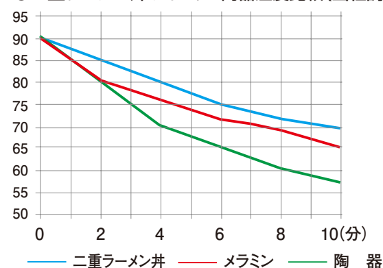
●二重ラーメン丼・メラミン・陶器温度比較(当社調べ)
